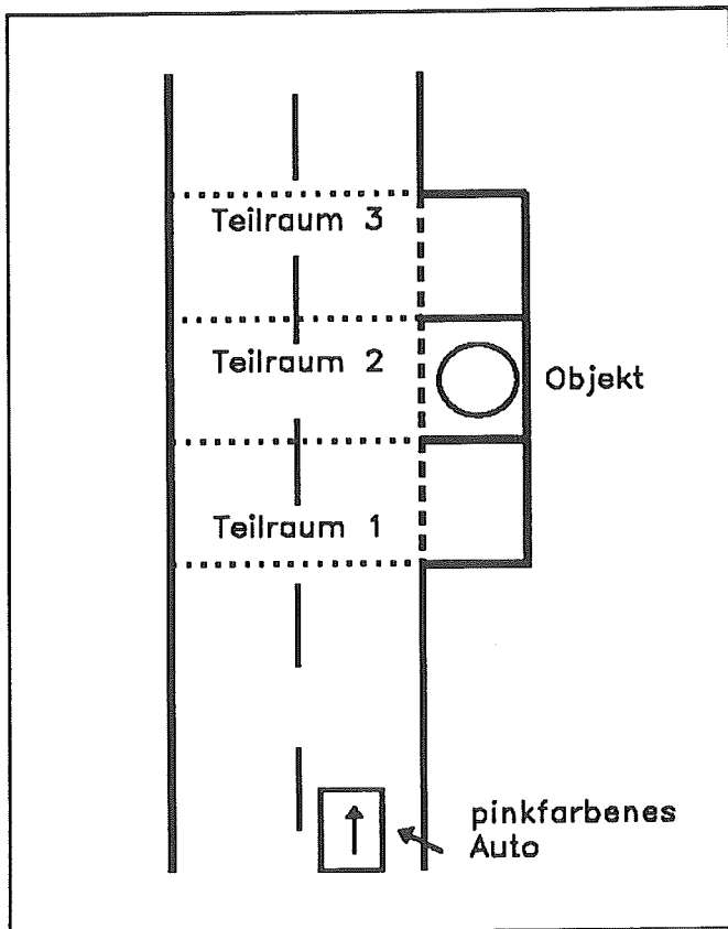
Abb.1: Teilräume im eindimensionalen Raum
